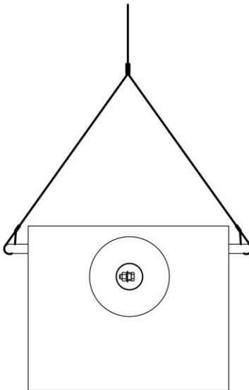
Рисунок Б.1 – Схема строповки трансформаторов мощностью 1,25; 2; 2,5; 4 кВ·А.
