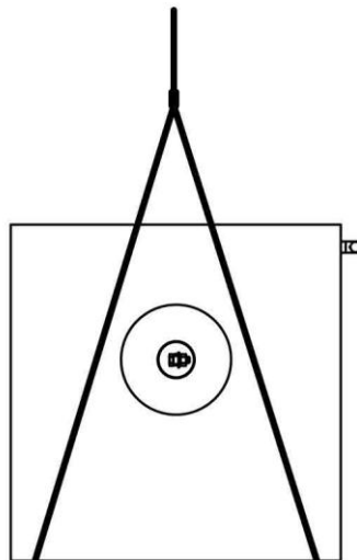
Рисунок Б.1 – Схема строповки трансформаторов мощностью 4; 6,3 и 10 кВ·А.
