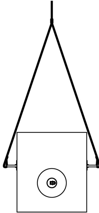
Рисунок Б.1 – Схема строповки трансформаторов мощностью 1,25; 2; 2,5 кВ·А.
